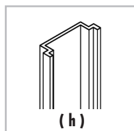
Profilé de jonction pour profilés de châssis à profilés de châssis avec vis autotaraudantes
