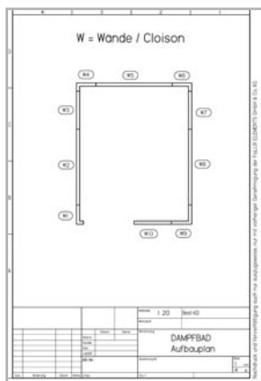
[DE] – Aufbauplan (Beispiel) [EN] – Plan of procedure (Example) [FR] – Schéma de montage (Exemple) [NL] – Montageschema (Voorbeeld)
